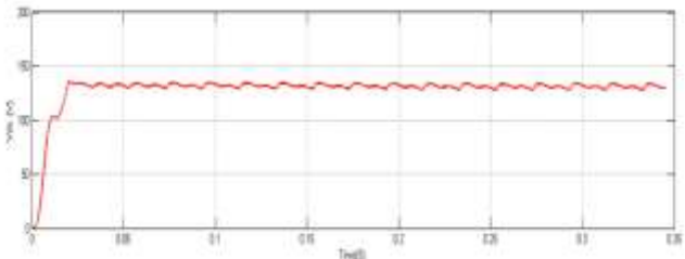
Fig. 9. DC link voltage.
